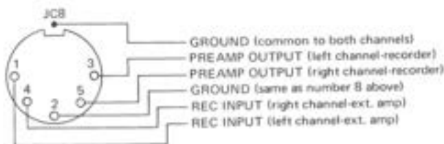
Front View of DIN JACK
