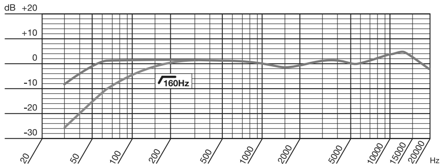
Réponse en fréquence C214
