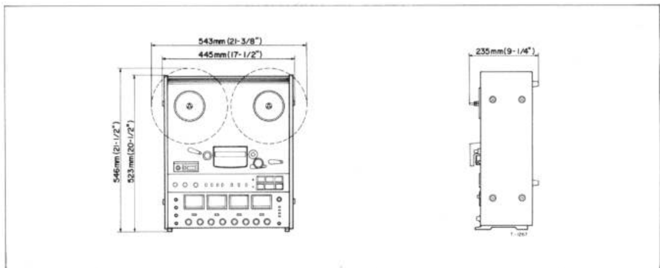
Fig. 2-1 Dimensions
