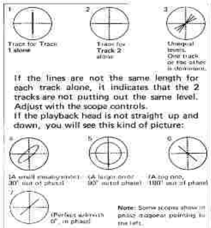
Fig. 2-23 Phase Shift
